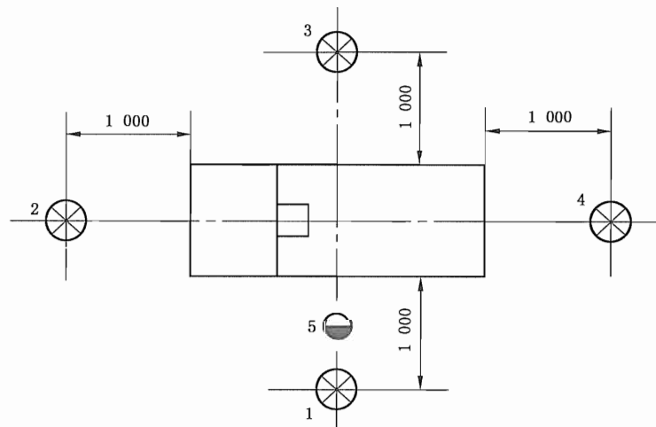
图 B.1 普通车床噪声测量点位置示意图
